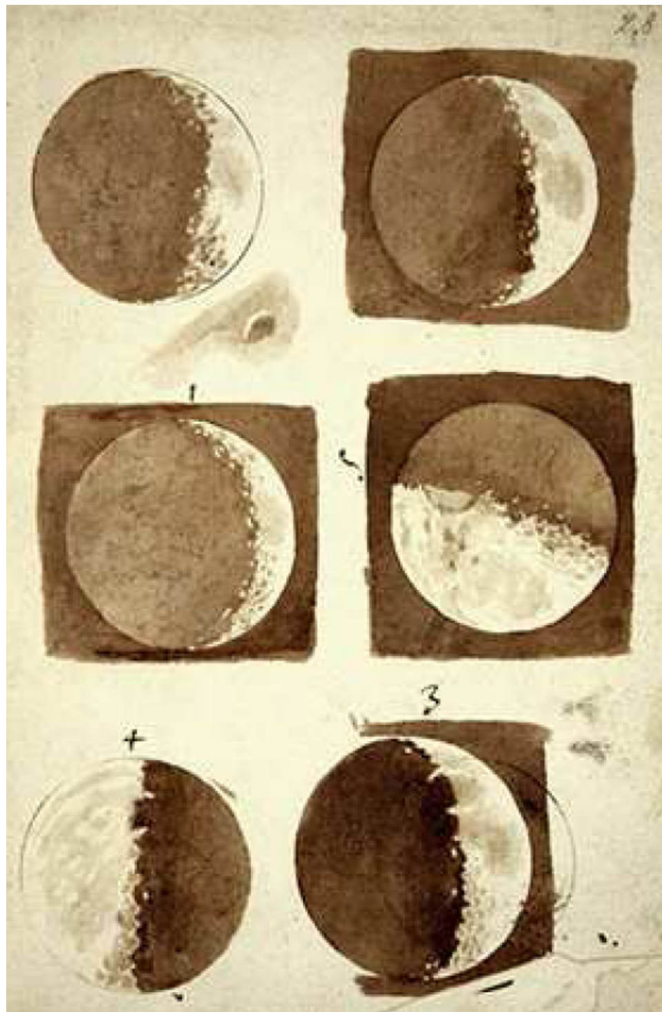
Fig.2.3 La superficie della Luna "disuguale, aspra, disseminata di cavità e sporgenze, non diversamente dalla faccia della Terra" [1].
